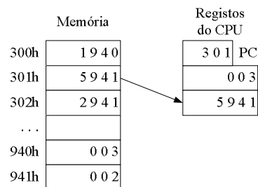
Figura 1.12 – Passo 3: Fetch da instrução Add
