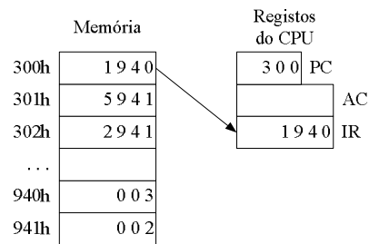
Figura 1.10 – Passo 1: Fetch da instrução Load 1
