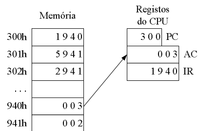
Figura 1.11 – Passo 2: Execução da instrução Load
