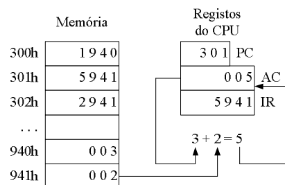
Figura 1.13 – Passo 4: Execução da instrução Add
