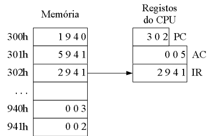
Figura 1.14 – Passo 5: Fetch da instrução Store
